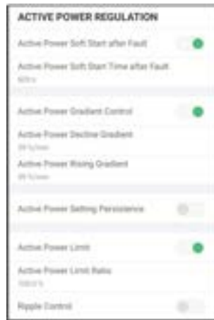
Abbildung 8-18 Regelung Wirkleistung
