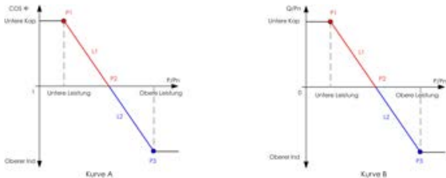
Abbildung 8-3 Q(P)-Kurve
