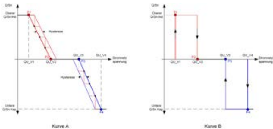
Abbildung 8-4 Q(U)-Kurve
