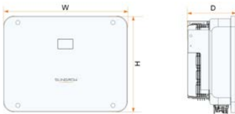
Abbildung 2-2 Abmessungen des Wechselrichters
